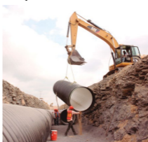
Figura 9. Bajado con maquinaria de tubería a la zanja, usar dos puntos de sujeción.
