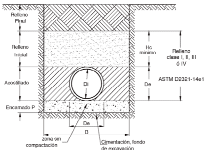
Figura 3. Sección de zanja típica para tuberías corrugadas de polietileno y polipropileno, conforme a norma ASTM D2321-20
