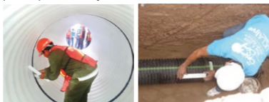
Figura 13. Verificación de posición de empaques con lana plástica por el interior y exterior.
