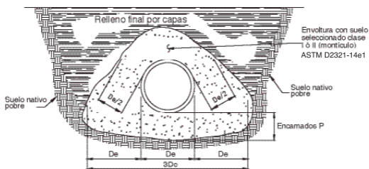
Figura 4. Sección de zanja típica para tubería de polietileno y polipropileno, cuando el suelo nativo no puede sostener un corte vertical cuando se instala en condición de terraplén
