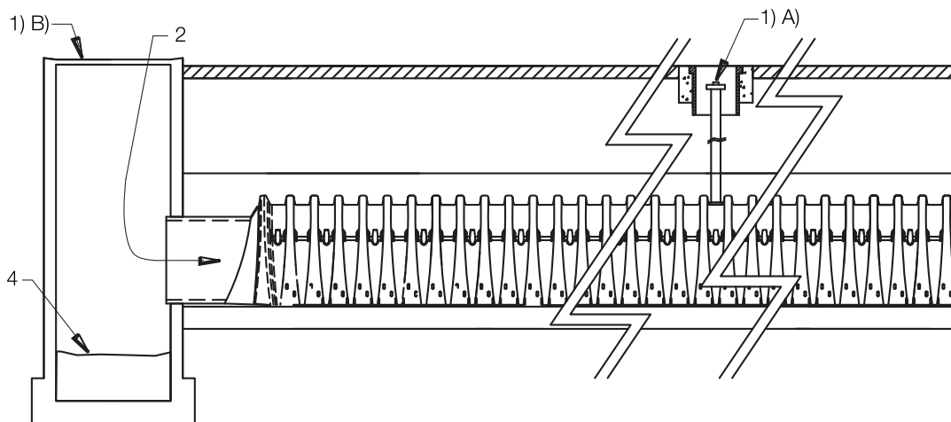
Hilera Aisladora de StormTech® (no a escala)
